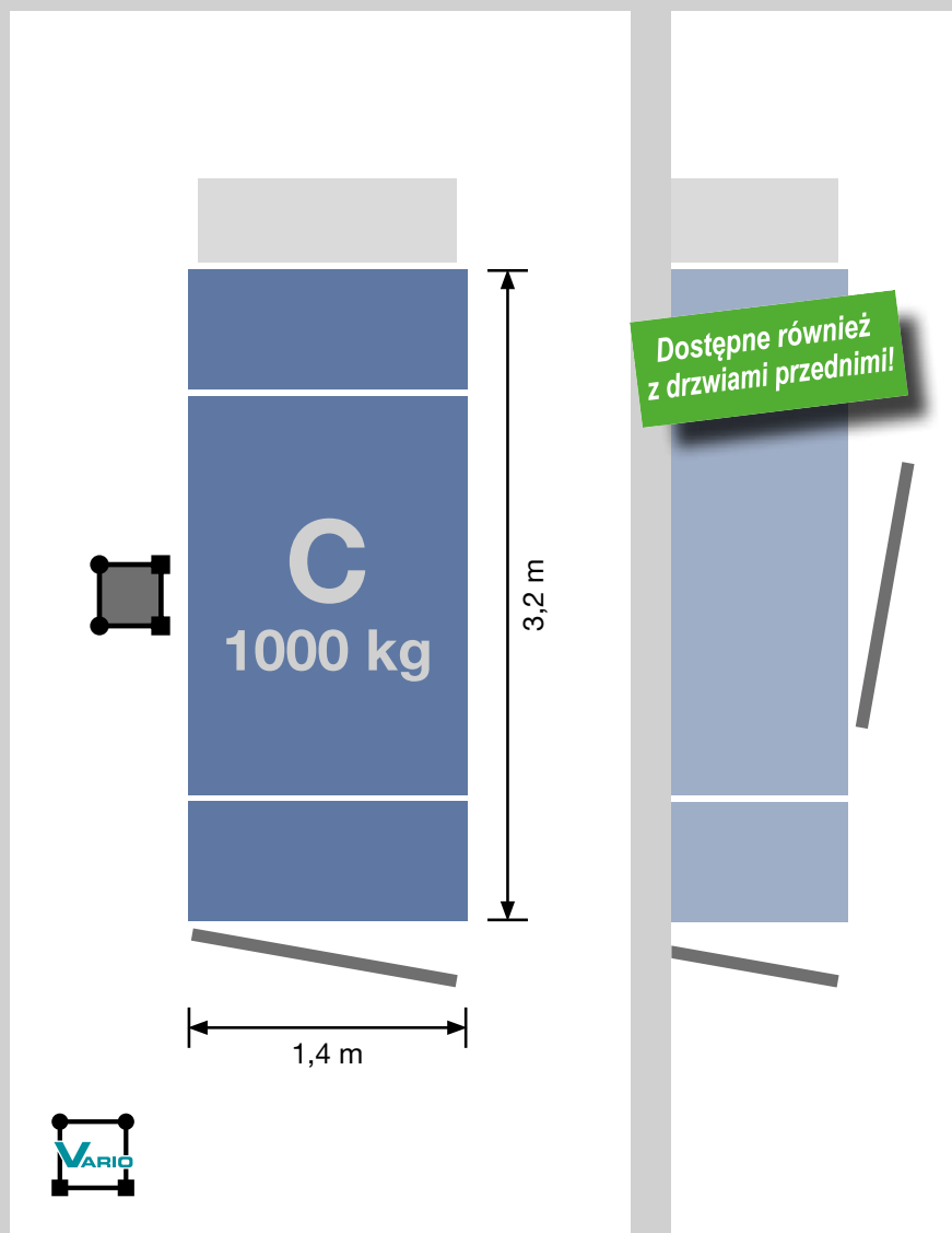
GEDA 1200 Z/ZP platforma C 1 drzwi ładunkowe / 1 rampa wyładownicza
