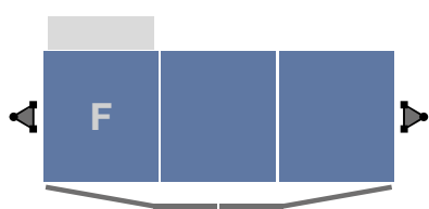
GEDA 1500 Z/ZP platforma H 2 x drzwi załadunkowe / 2 rampy wyladowcze
