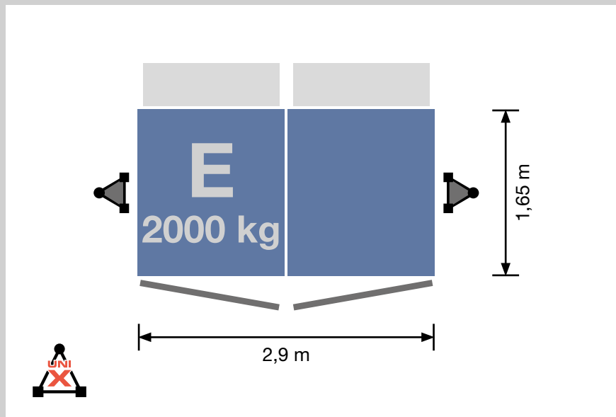
GEDA 1500 Z/ZP platforma E 2 x drzwi ładunkowe / 2 rampy wyładownicze
