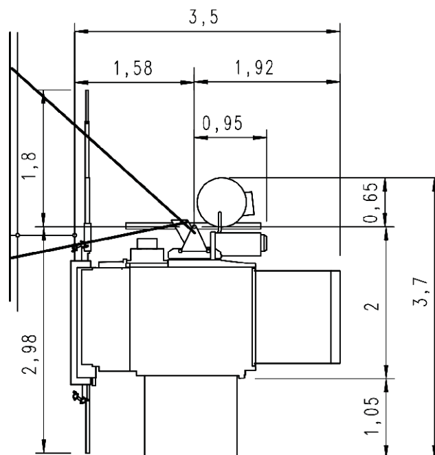
Normalne zapotrzebowanie na miejsce przed rusztowaniem
