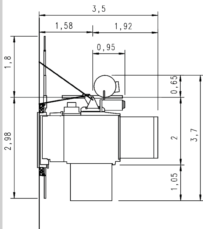
Normalne zapotrzebowanie na miejsce przed ścianą
