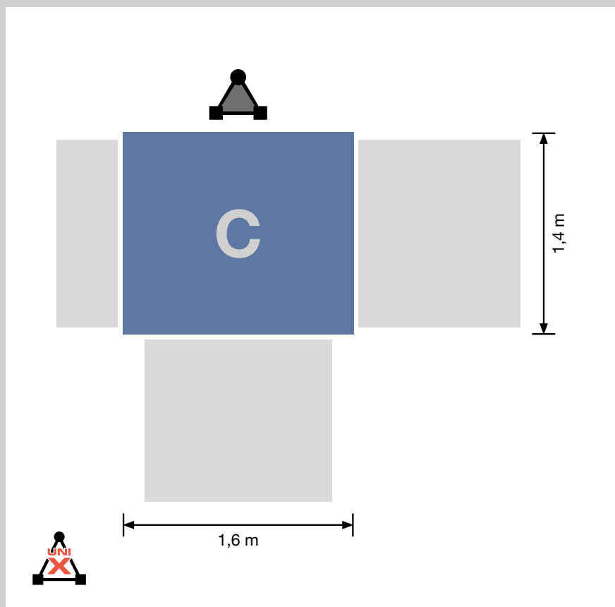
GEDA 500 Z/ZP platforma C 2 rampy załadunkowe / 1 rampa rozładunkowa
