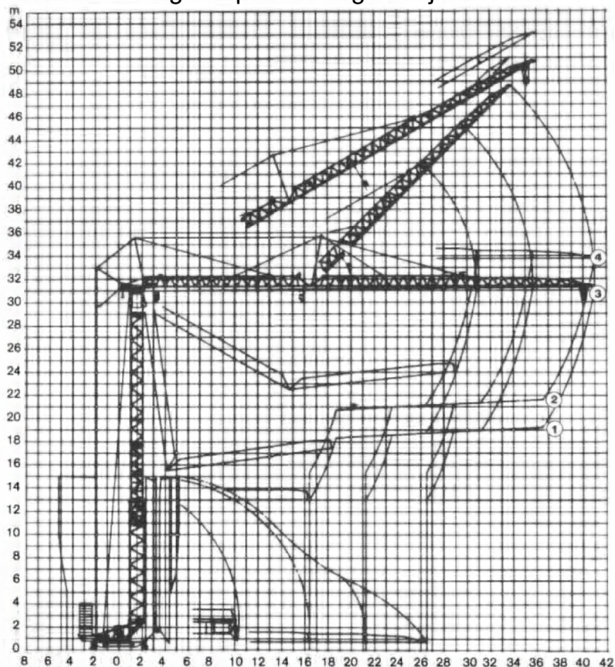
Montaż - diagram potrzebnego miejsca
